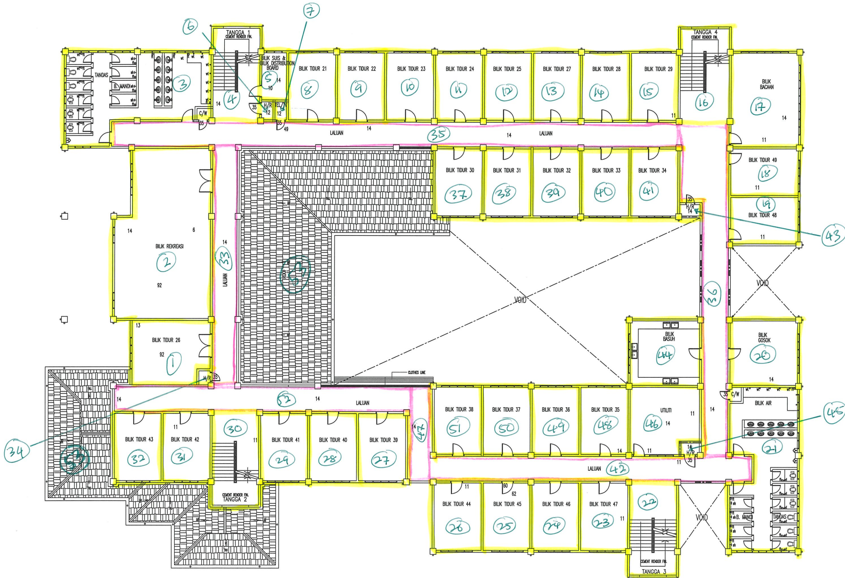
ASRAMA PEREMPUAN D - PELANLANTAI ARAS SATU
